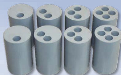
孔径 66mm (4帯水層対応) の遮水栓
