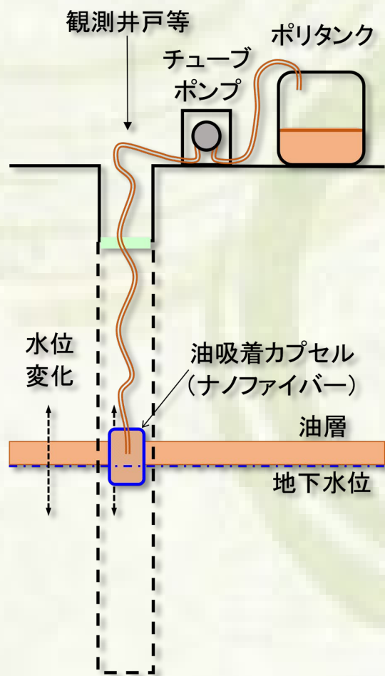
孔内油層回収装置の概要
