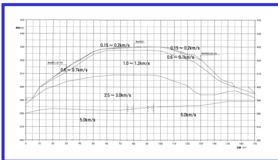
既存のハギトリ法解析結果
