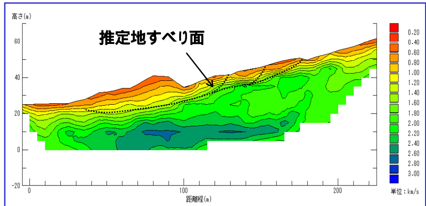
高密度弾性波探査結果
