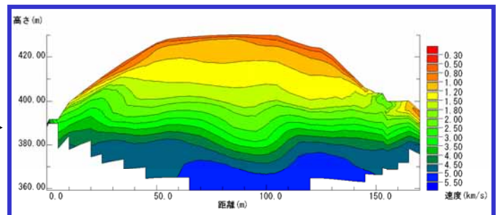
高密度弾性波探査による再解析結果(速度分布図)
