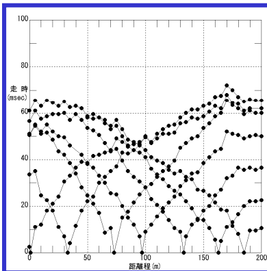
既存の走時データ
