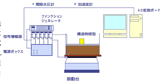
図1 振動台実験システム模式図
