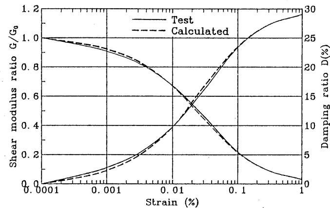
図-4 拘束圧 0.5 \rightarrow 0.25\text{ kg/cm}^2
