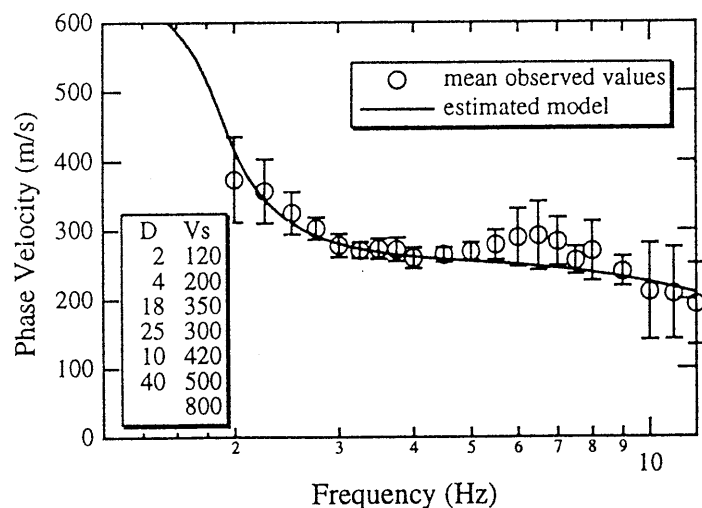
図-3 KMBにおける位相速度分散曲線
