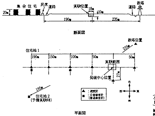
図-1 現場概要および計測器配置図
