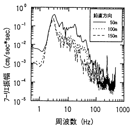
図-3 地表面速度フーリエスペクトル (上下動、1孔、装薬箇所1カ所、装薬量3kg)
