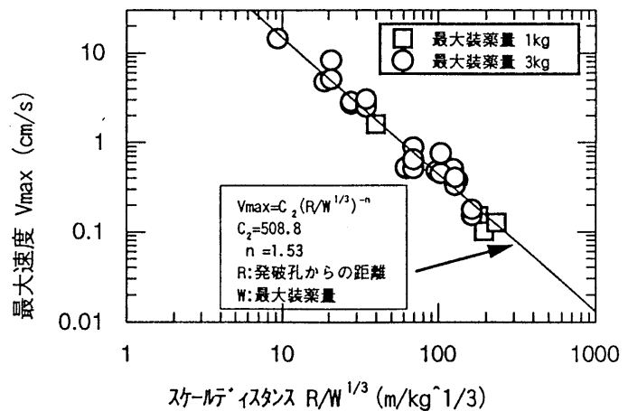
図-4 地表面速度の距離減衰（上下動）
