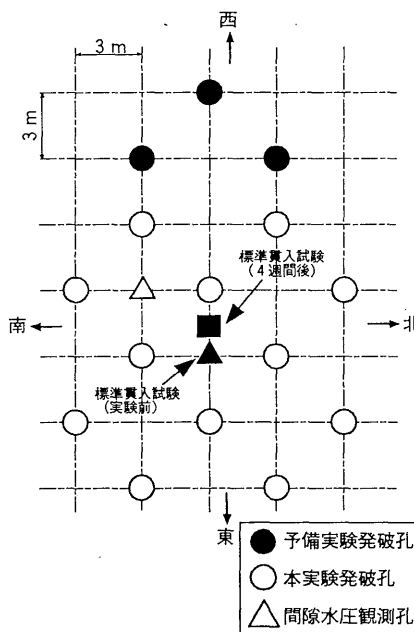
図-1 標準貫入試験位置
