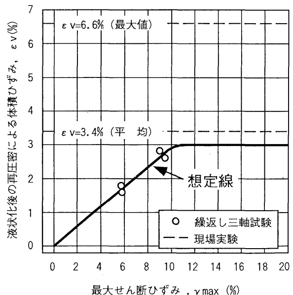
図-4 液状化後の \epsilon_v \sim \gamma_{max}
