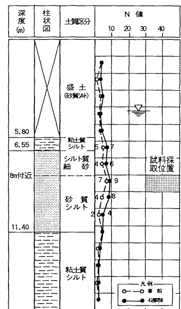
図-2 N値の分布
